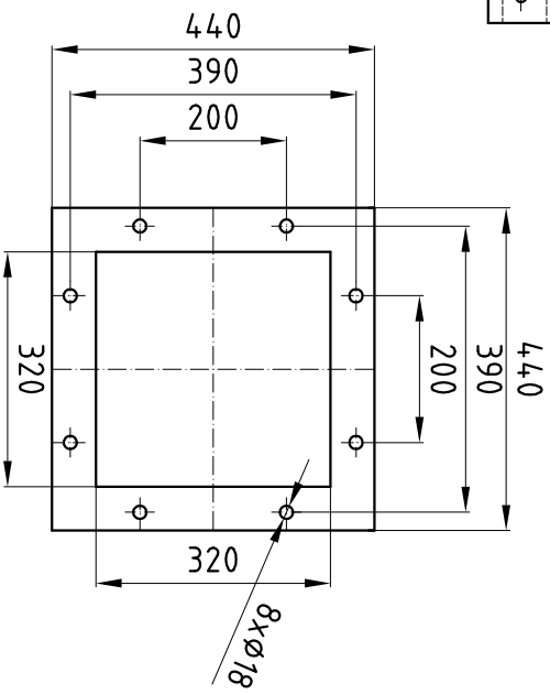
PŘÍRUBA "A"
